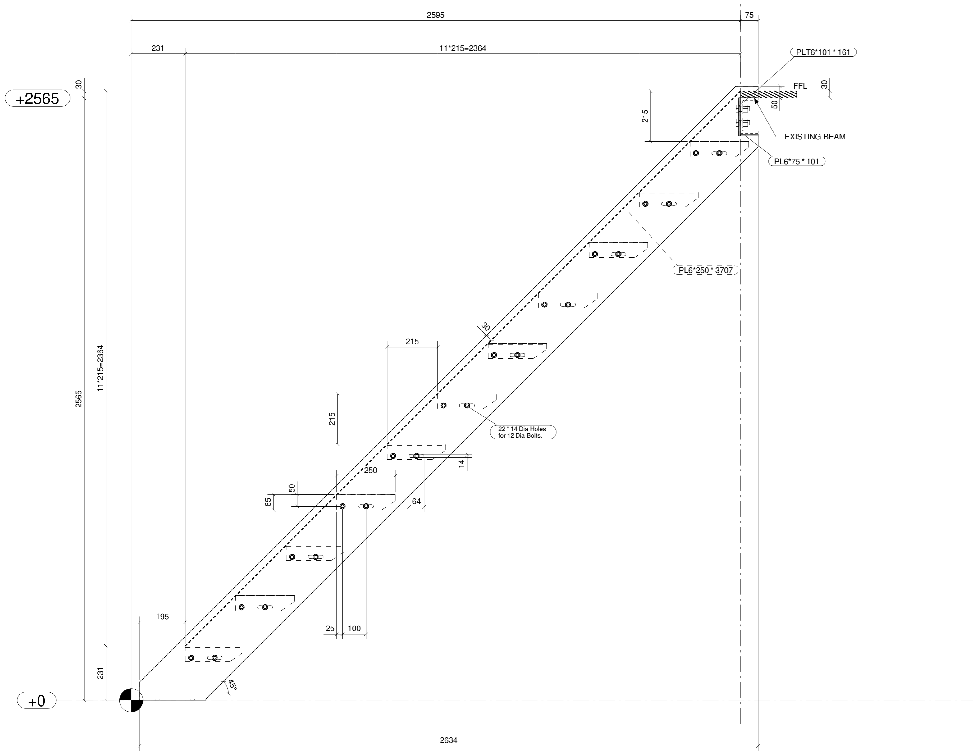
A-A 1:10
